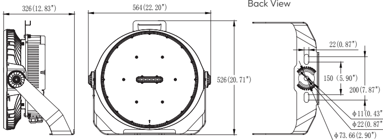
Technical Drawing: 12.83" (D) x 22.2" (W) x 20.71" (H)
