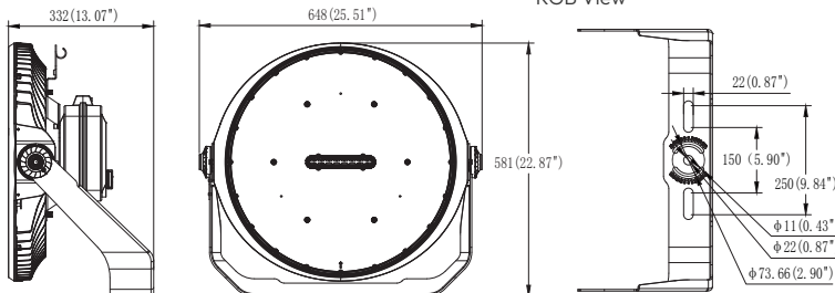
Technical Drawing: 13.07" (D) x 25.51" (W) x 22.87" (H)
