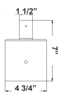
DAB-PA4-1 4 3/4"(W) x 7"(H)
