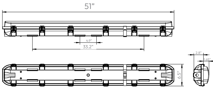
Technical Drawing: 51" (W) x 6.5" (H) x 4.45" (D)
