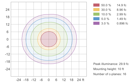
Iso-illuminance plot
