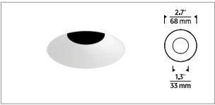
ROUND BEVEL
